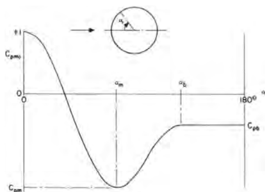
Figura C3.3.26 - Coefficiente di pressione esterna c_{pe0}
