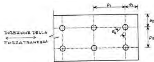
Figura C4.2.34 –Parametri significativi per i collegamenti
