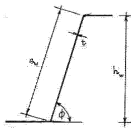
Figura C4.2.33 –Anime di profili sottili
