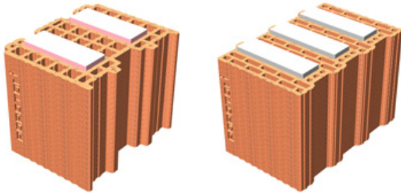
Fig. 3 – Mattoni con isolante: POROTON® ISO 30 e POROTON® ISO 36.
